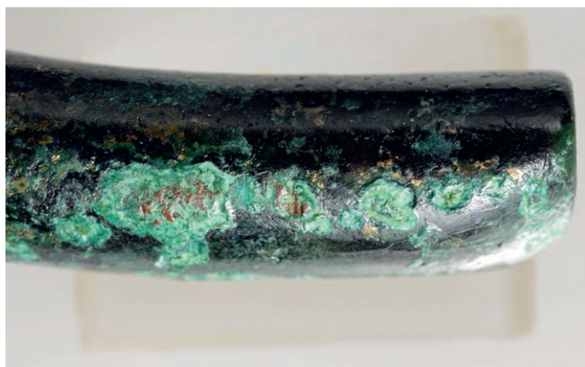
Abb. 6. Wagenhausen TG Etwilwil, Tättbühl. Lochfrass im Armreif Kat.-Nr. 4. Foto AATG, L. Leuenberger.
