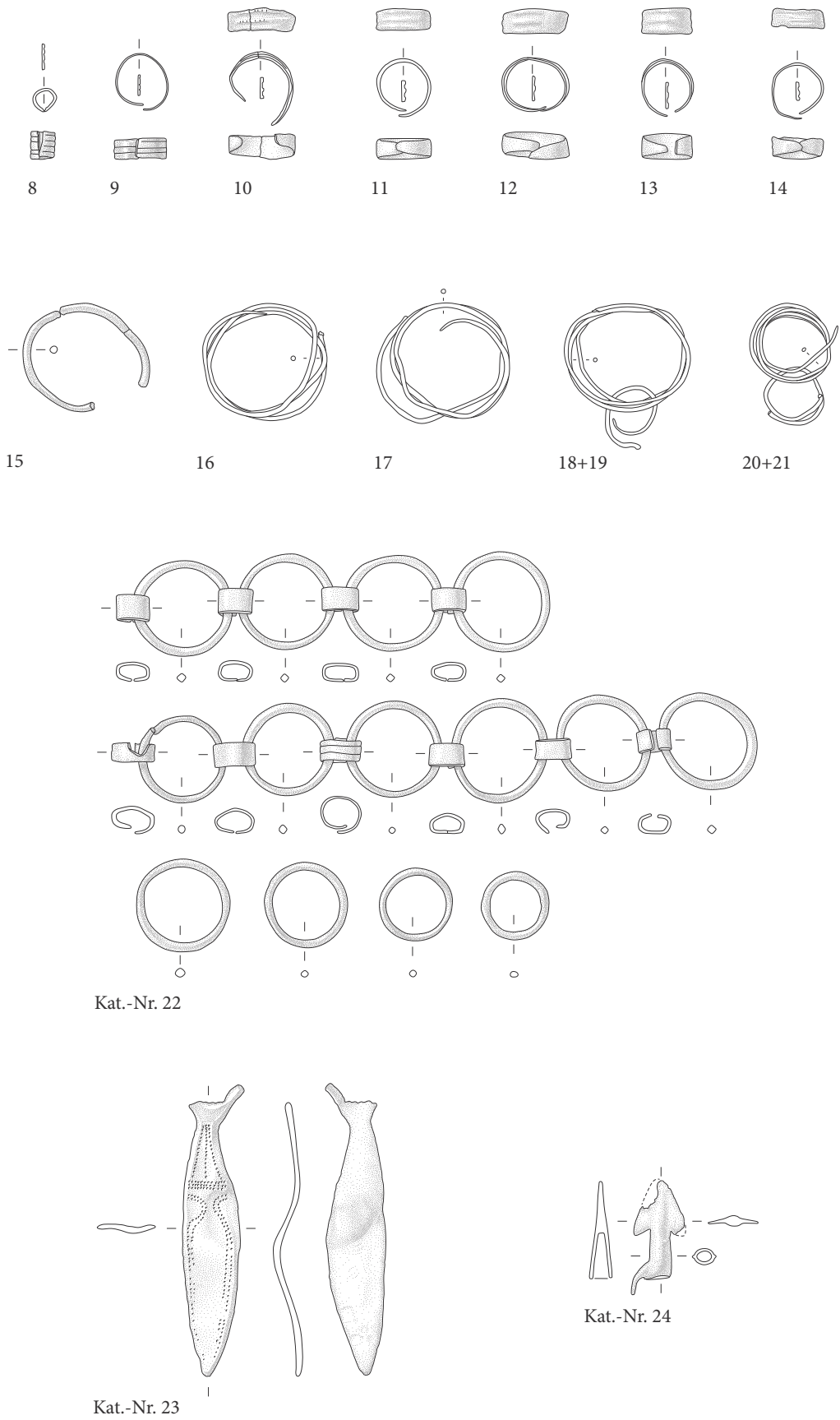
Abb. 16. Wagenhausen TG Etzwilen, Tättebüel. Blechhülse, Fingerringe, Drahtring, Drahtspiralen, Ringkette, lanzettförmiger Anhänger und Tüllenpfeilspitze. M. 1:2. Zeichnung AATG, J. Näf.
