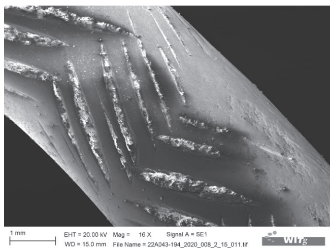
Abb. 8. Wagenhausen TG Etzwilen, Tättbüel. REM-Aufnahme mit Ausschnitt der Tannenzweig-Verzierung von Armring Kat.-Nr. 3. Foto WITg, T. Bogatzky.
